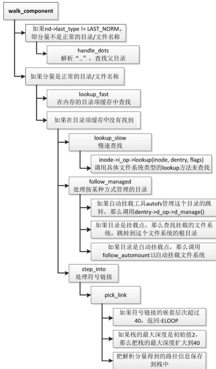
图6.20 函数walk_component的执行流程
