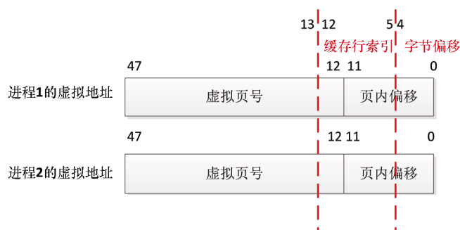
图3.150 VIPT缓存的别名问题
