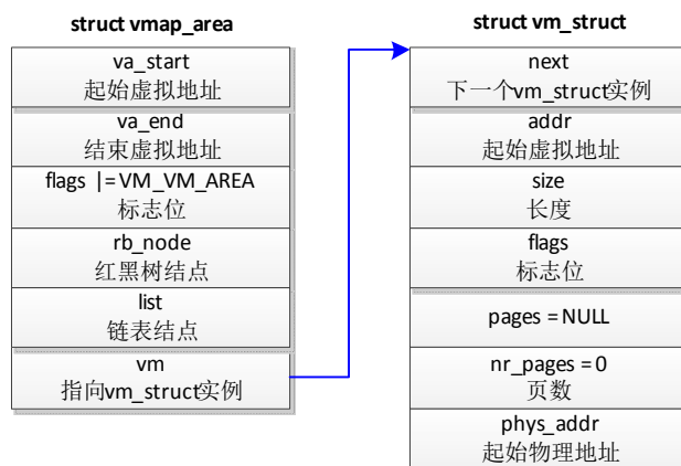
图3.47 使用vmap函数分配虚拟内存区域
