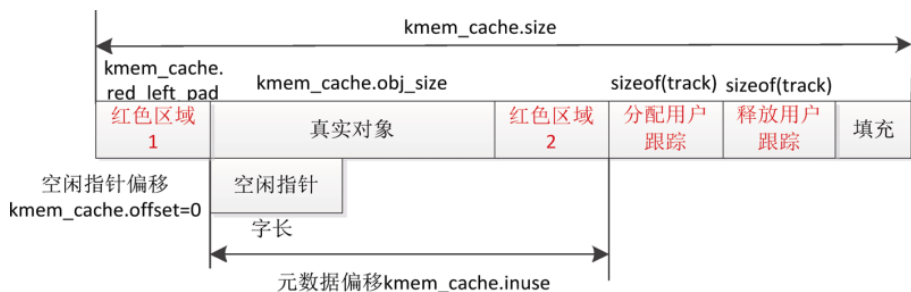
图3.39 空闲指针重用真实对象的第一个字
