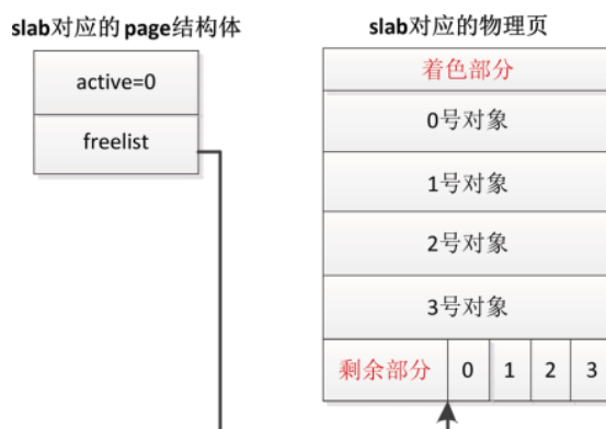
图3.32 把空闲对象链表放在slab尾部
