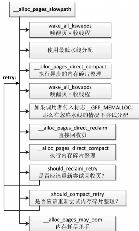
图3.20 慢速路径
