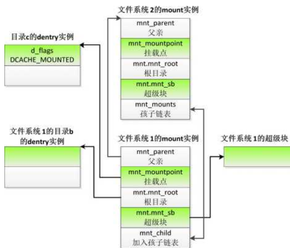
图6.9 绑定挂载
