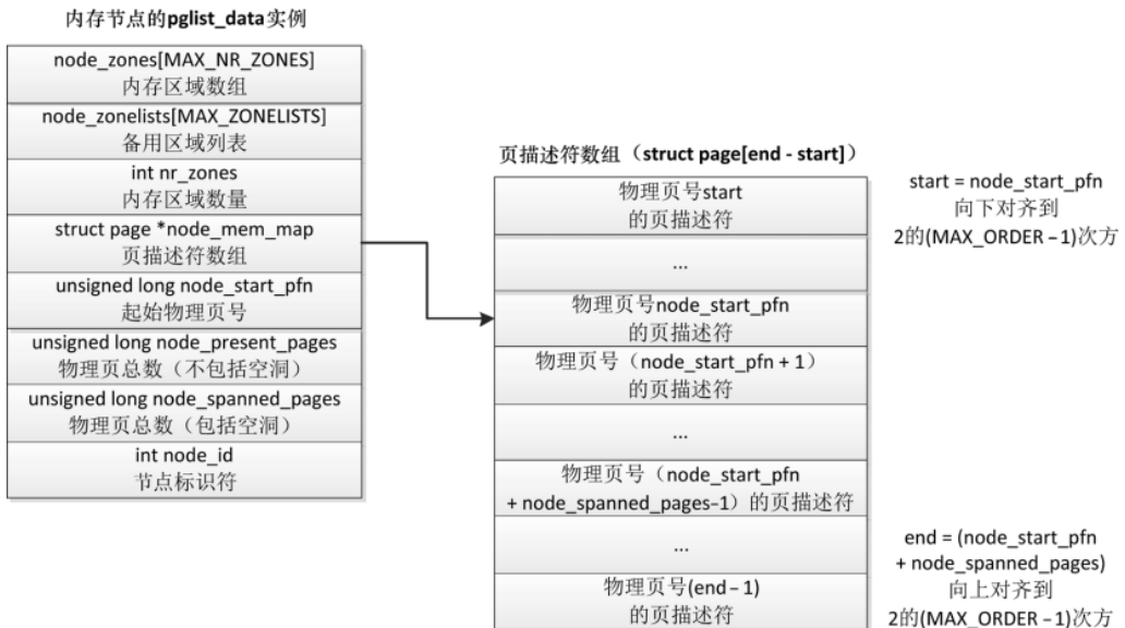
图3.16 内存节点的 pglist_data 实例
