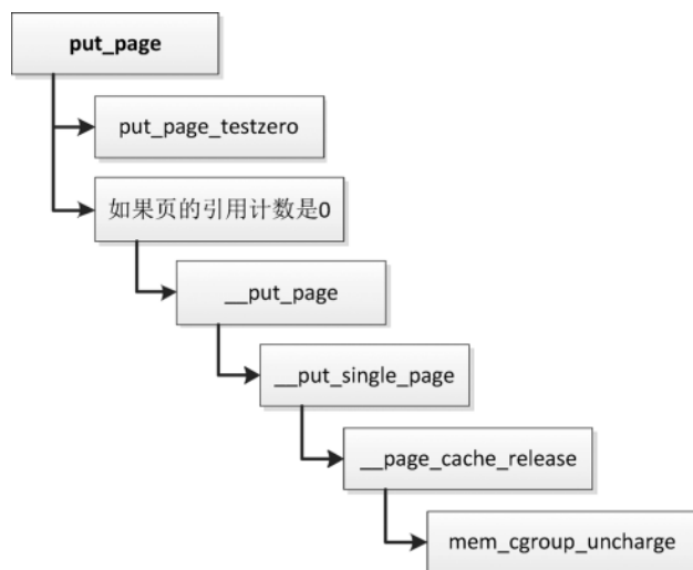
图3.138 释放页时撤销内存记账
