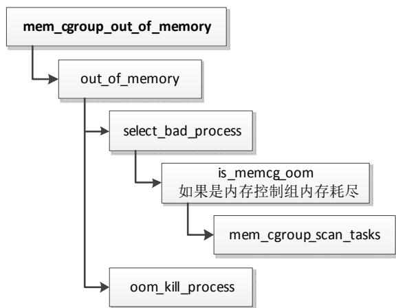
图3.147 函数 mem_cgroup_out_of_memory 的执行流程
