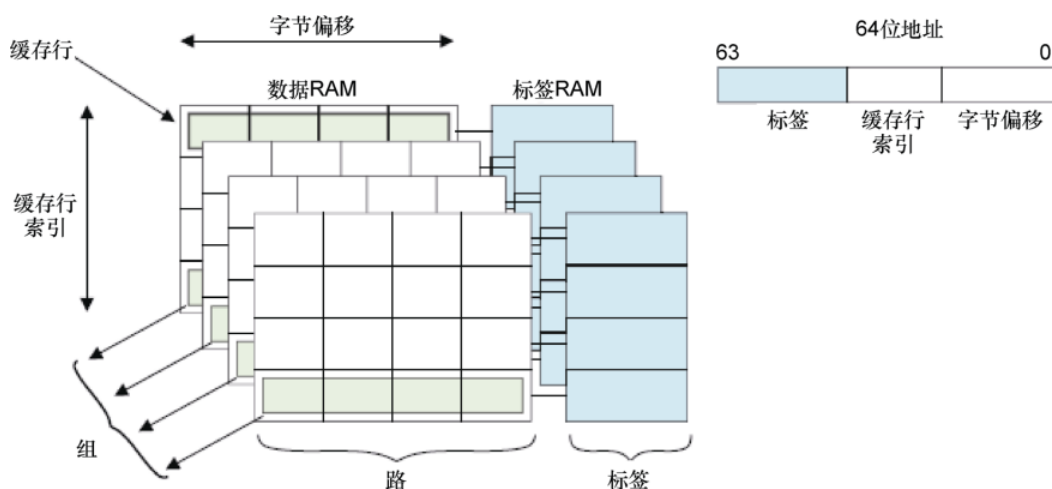
图3.149 缓存的结构
