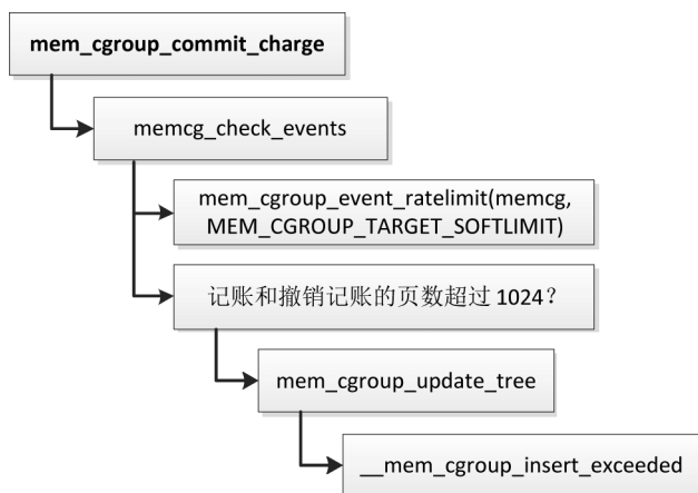
图3.141 检查软限制
