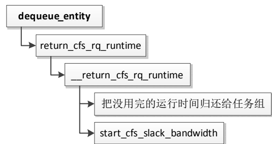
图2.36 公平运行队列归还运行时间
